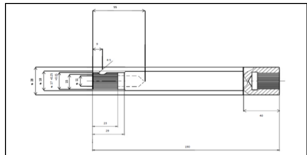
A01-16) Axe biplace (L=190 mm) Biplace shaft (L=190 mm)
